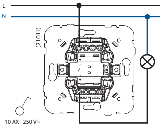
JEDNOPOLNI PREKIDAČ
