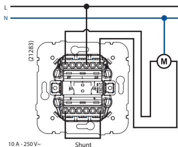
VENECIJANSKI DUPLI TASTER SA VIŠE POLOŽAJA ZA KONTROLU ROLETNI (kontrola sa 1 tačke)
