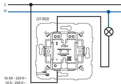
GREBENASTI PREKIDAČ 16 A PREKIDAČ SA KANAPOM
