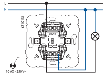
JEDNOPOLNI PREKIDAČ SA KONTROLNOM LAMPOM
