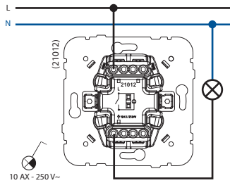
JEDNOPOLNI PREKIDAČ SA LED SVETLOM
