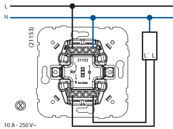
TASTER PREKLOPNIK SA NEZAVISNOM KONTROLNOM LAMPOM
