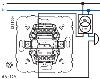
TASTER PREKLOPNIK SA INDETIFIKACIJOM 12 V
