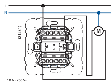
VENECIJANSKI DUPLI TASTER
