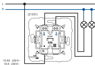
DVOSMERNI PREK. SA KLJUČEM TASTER SA KLJUČEM
