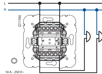
DUPLI TASTER
