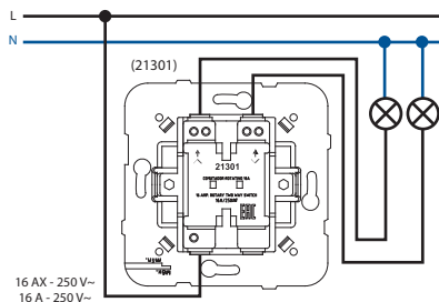
GREBENASTI DVOSMERNI PREKIDAČ 16 A GREBENASTI TASTER
