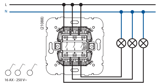
PREKIDAČ SA TRI KOLA
