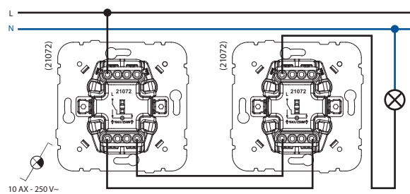
DVOSMERNI PREKIDAČ SA LED SVETLOM
