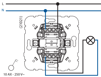
DVOPOLNI PREKIDAČ
