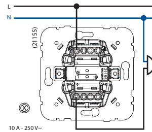
TASTER PREKLOPNIK SA INDETIFIKACIJOM 250 V
