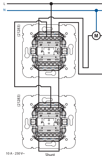
VENECIJANSKI DUPLI TASTER SA VIŠE POLOŽAJA ZA KONTROLU ROLETNI (Kontrola sa 2 ili više tačaka)
