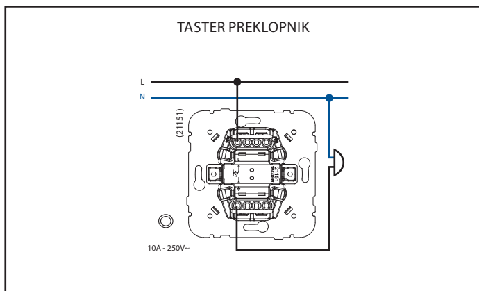
TASTER PREKLOPNIK SA LED SVETLOM - 250 V
