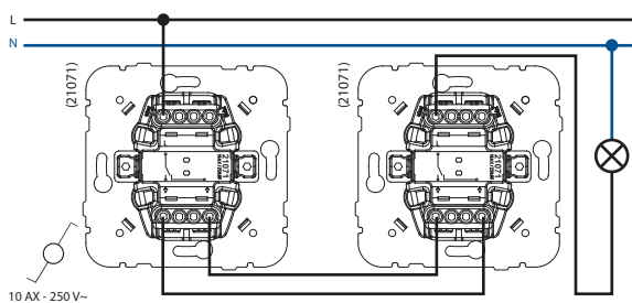
DVOSMERNI PREKIDAČ - 10 A i 20A
