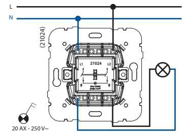
DVOPOLNI PREKIDAČ SA KONTROLNOM LAMPOM - 20 A
